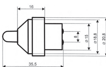
УПС2А
