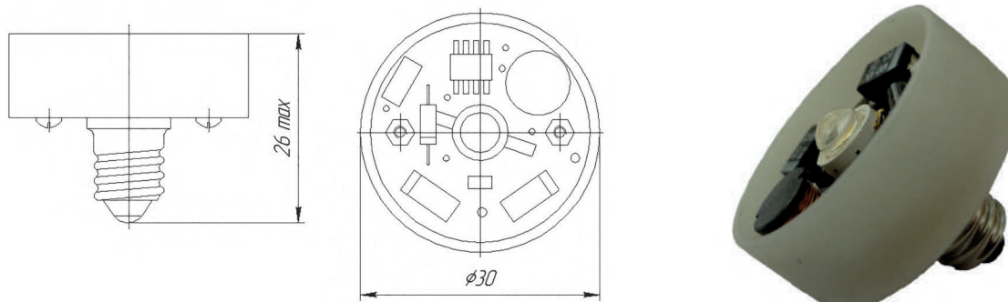
ЛАМПА-1
