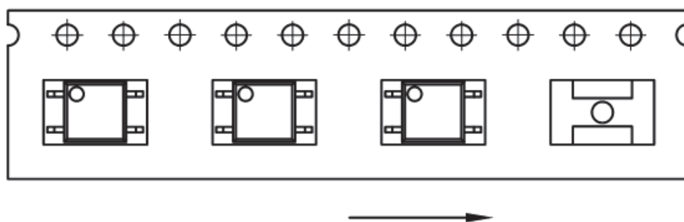
Чертеж упаковочной ленты для микросхем и оптопар в корпусах SOP4 с указанием ориентации выводов корпуса
