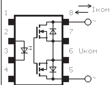
Схема включения Б:
