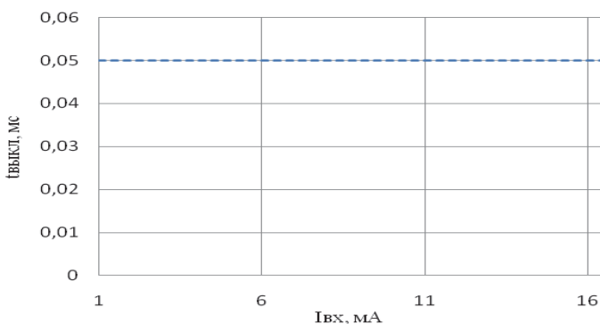
Зависимость времени выключения от входного тока ( I_{вх} = 5 \text{ мА} , U_{ком} = 50 \text{ В} , R_n = 1000 \text{ Ом} )
