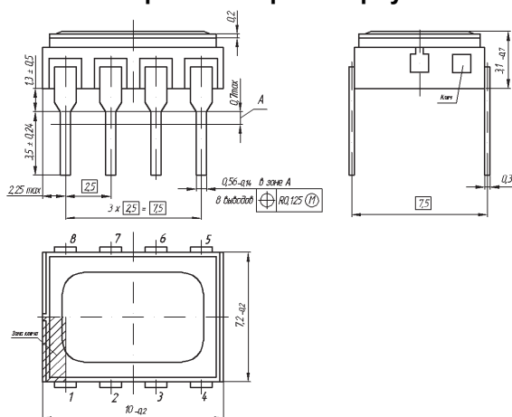
Габаритный чертеж корпуса
