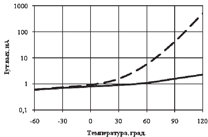
Диапазон значений тока утечки на выходе в закрытом состоянии в диапазоне температур
