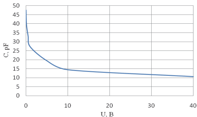
Зависимость выходной емкости от коммутируемого напряжения
