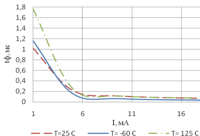
Зависимость времени включения от входного тока ( I_{вх} = 5 \text{ мА} , U_{ком} = 50 \text{ В} , R_n = 1000 \text{ Ом} )
