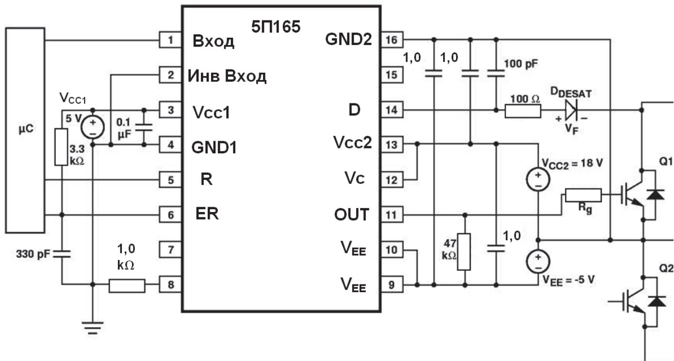
Рекомендуемая схема включения
