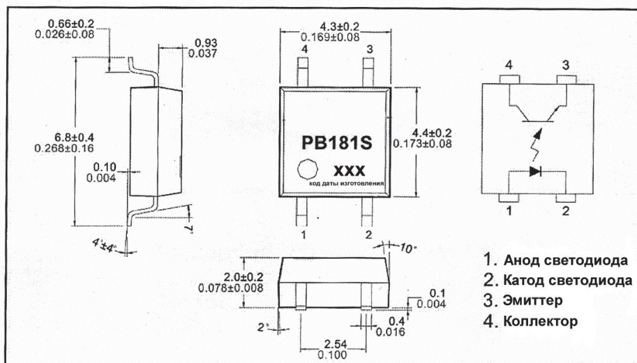
Габаритные и присоединительные размеры (мм/дюйм) Назначение выводов корпуса
