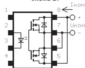
Схема Б:
