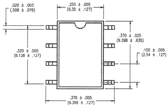
Вид сверху
