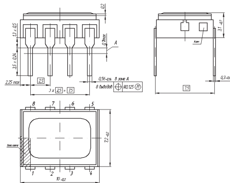
Габаритный чертеж корпуса и назначение выводов
