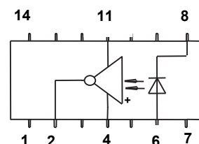
Электрическая схема
