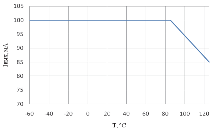
Зависимость максимального тока коммутации от температуры окружающей среды (при I_{вх} = 5 \text{ мА} )
