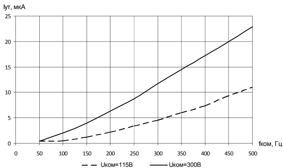
Типовая зависимость тока утечки в закрытом состоянии I_{\text{ут}} от частоты коммутируемого напряжения f_{\text{ком}}
