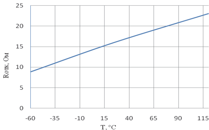
Зависимость сопротивления в открытом состоянии от температуры ( I_{вх} = 5 \text{ мА} , I_{вых} = 100 \text{ мА} )
