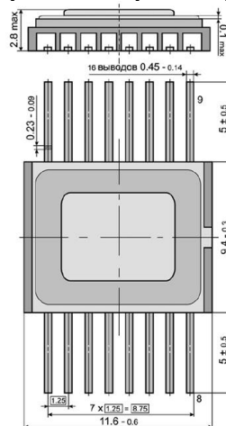
Габаритный чертеж корпуса
